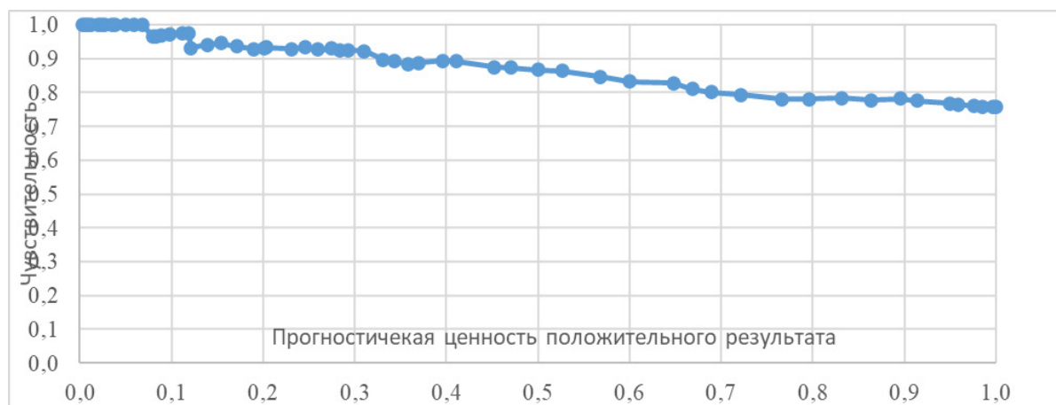
Рис. 2 – Кривая precision-recall
